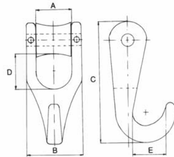
CHOKER HOOK
